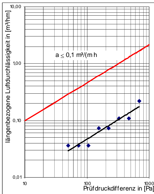
Diagramm 1 Längenbezogene Luftdurchlässigkeit bei Überdruck
