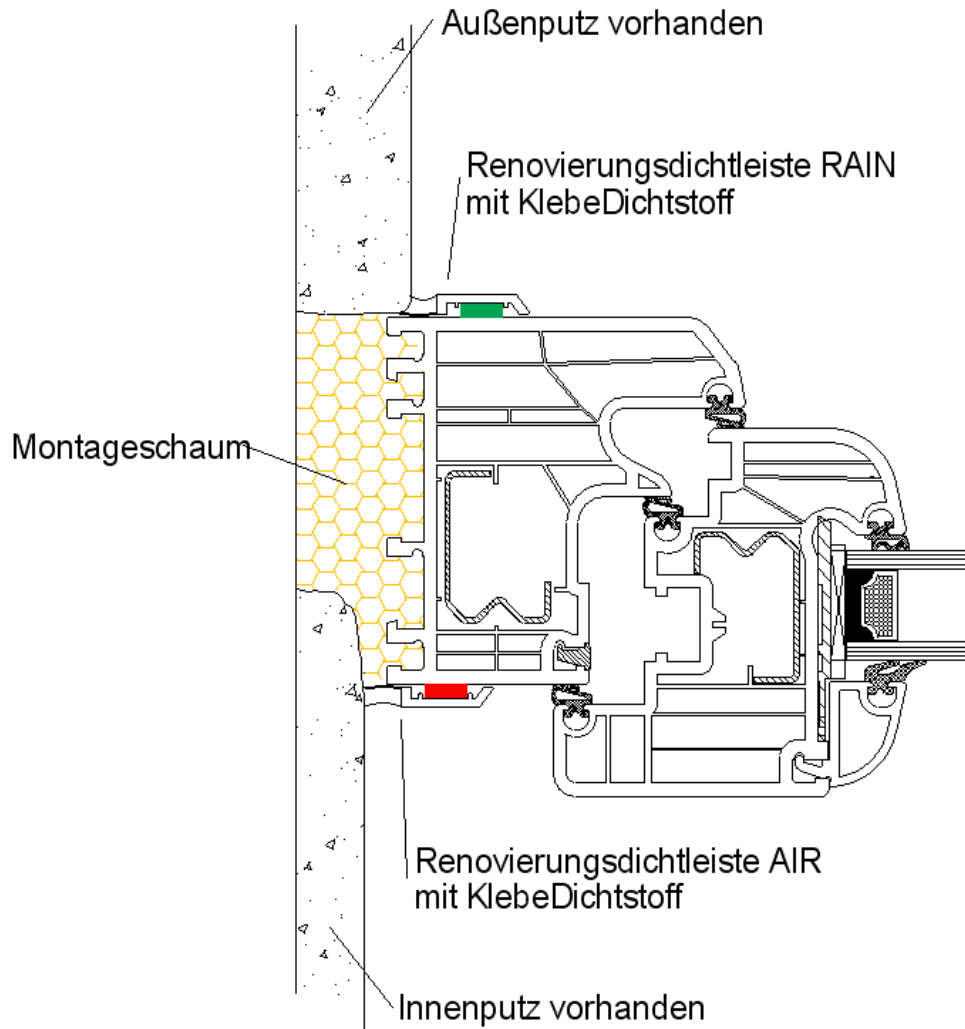
Bild 2 Seitliche und obere Anschlussausbildung
